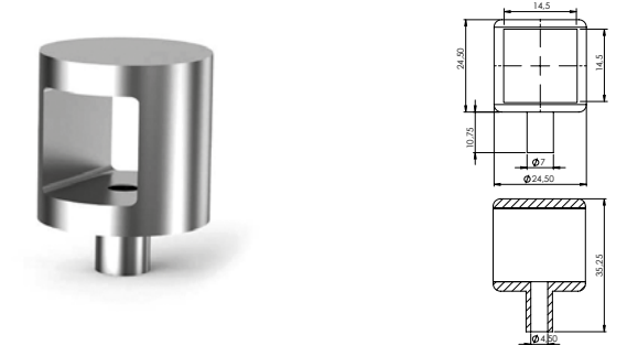
14x14 Emniyet Tutamağı
