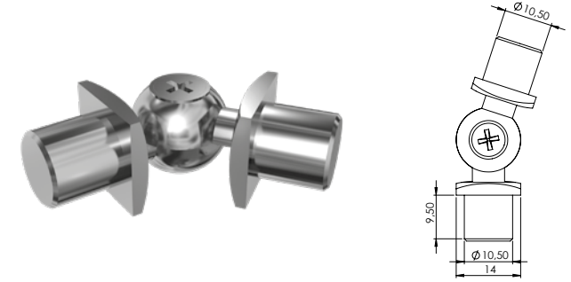
14x14 Emniyet Tutamağı
